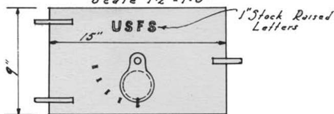
~ ELEVATION ~
