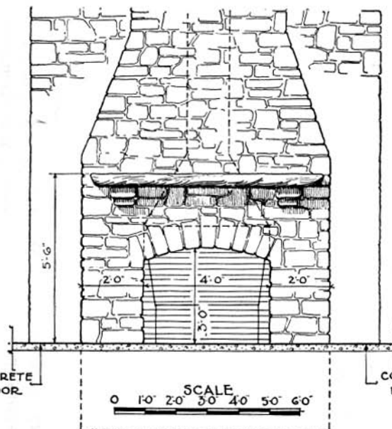
ELEVATION - FIG. 1
