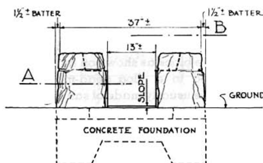
ELEVATION FIG. 2
