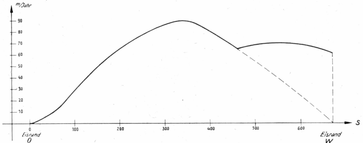
Abb. 1: Geschwindigkeitsprofil am Nisqually-Gletscher
