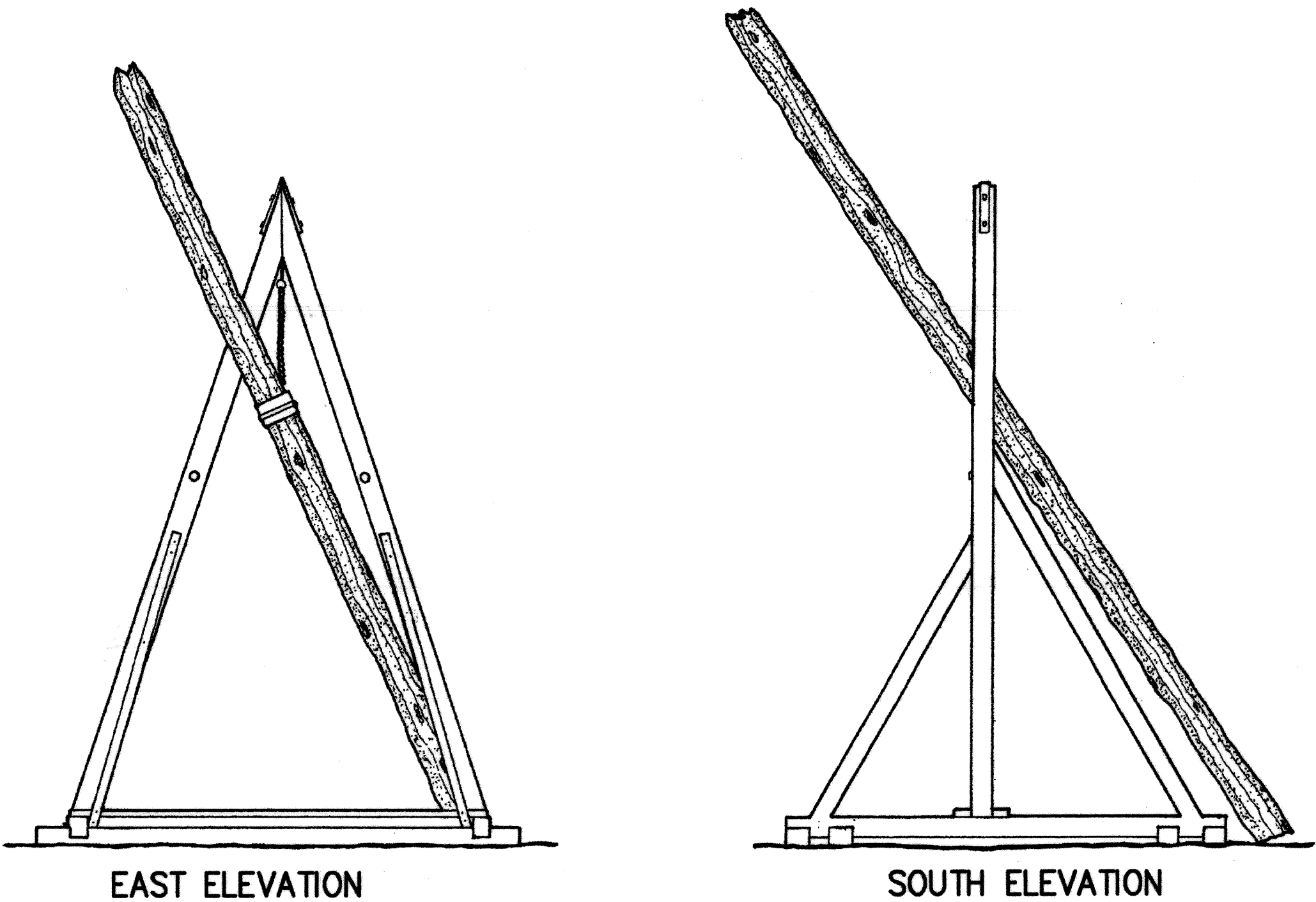
HAY DERRICK
