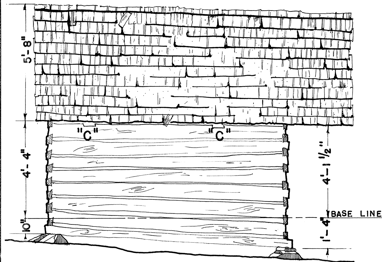
NE ELEVATION
