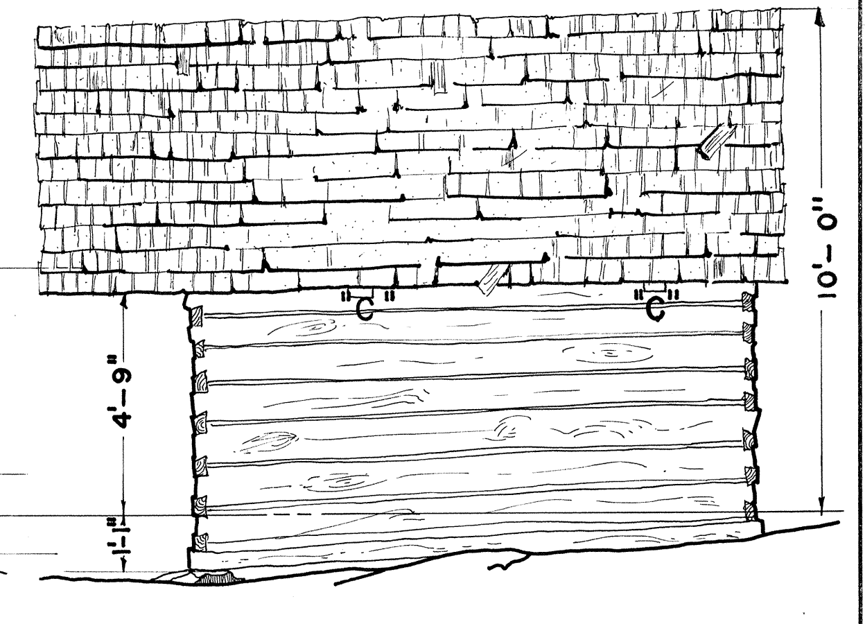
SW ELEVATION
