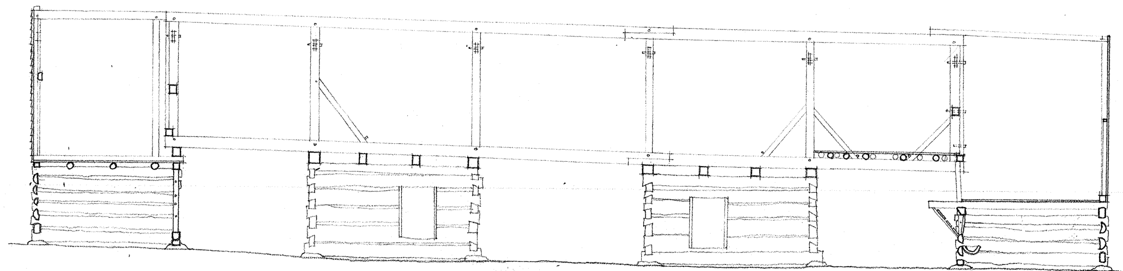
SECTION A-A
