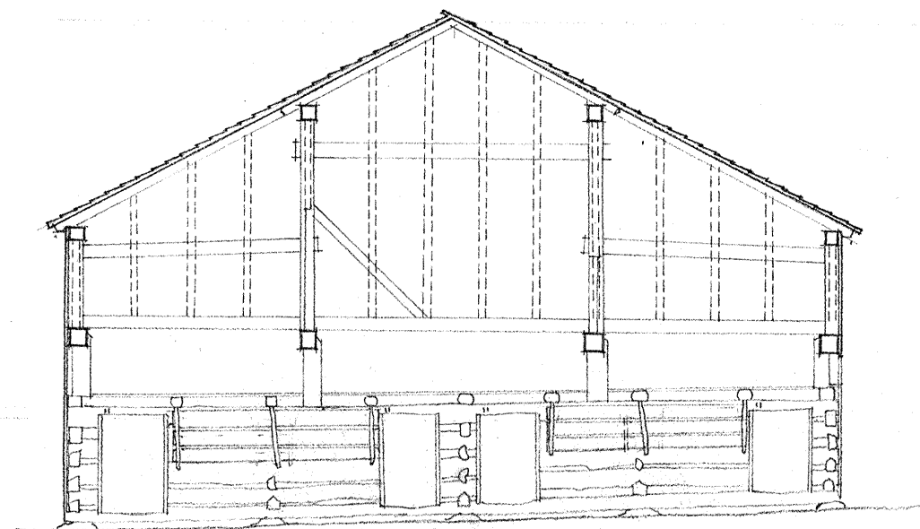
SECTION D-D
