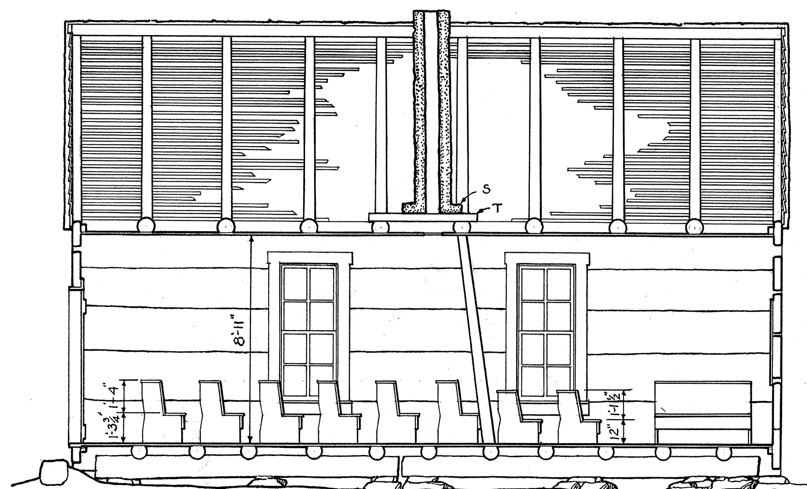
SECTION A-A
