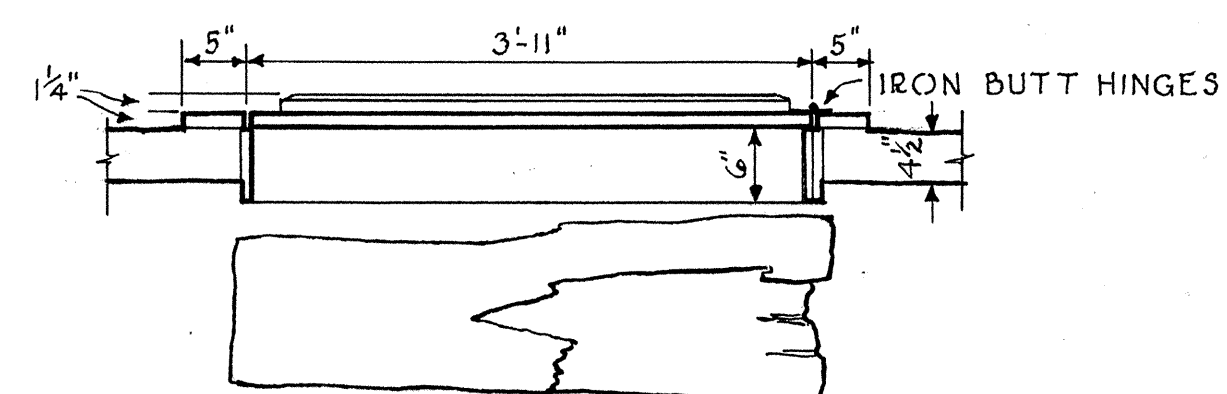
PLAN DOOR DETAILS
