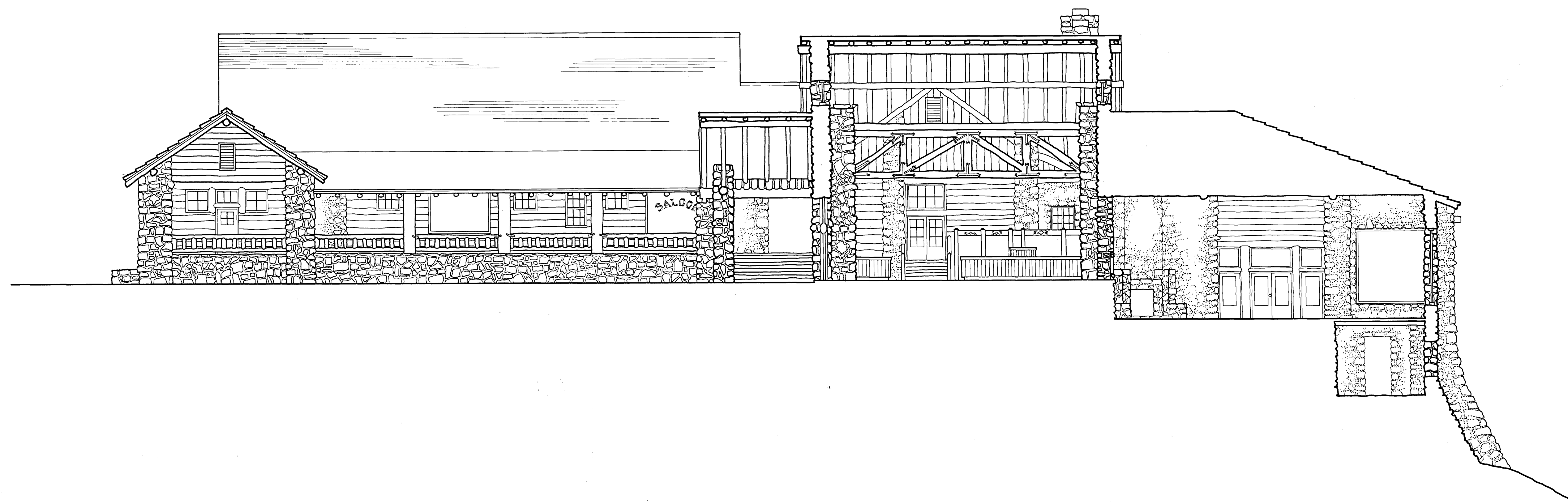
SECTION A-A
