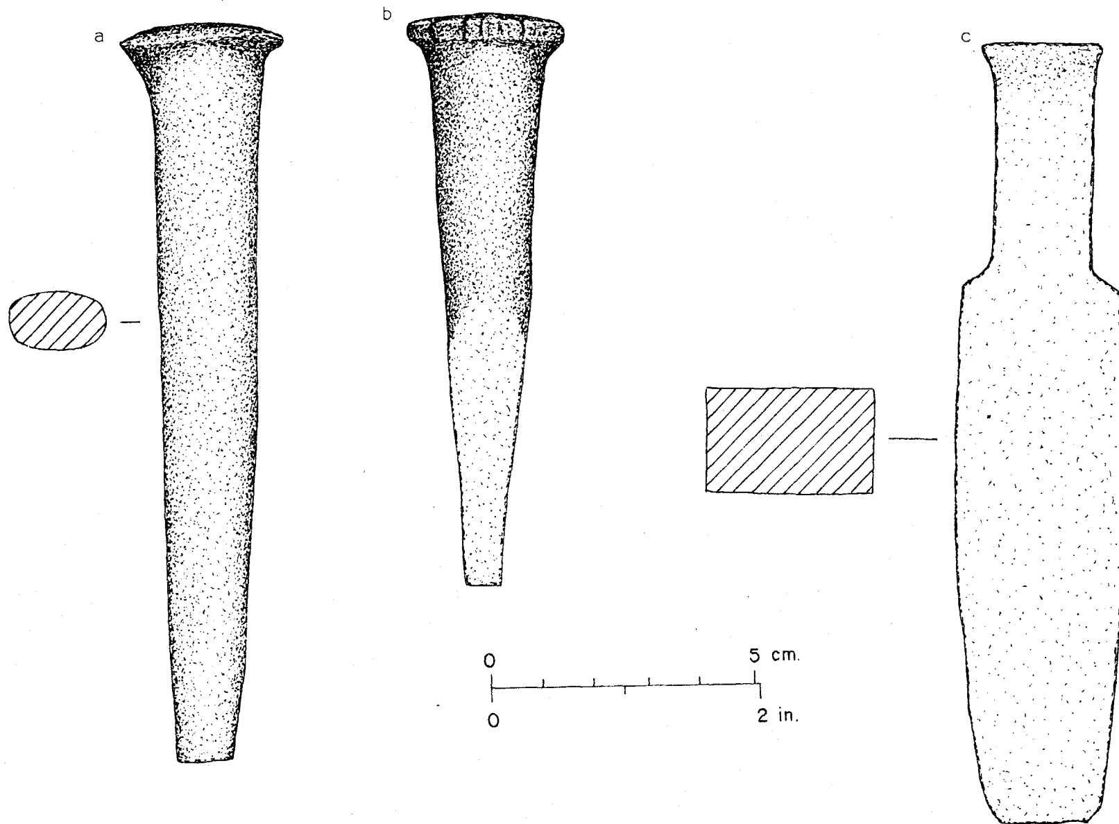
Fig. 125 -- Punches from F523: a). punch (FOVA 28263); b). punch (FOVA 27542) and c). punch (FOVA 28390).
