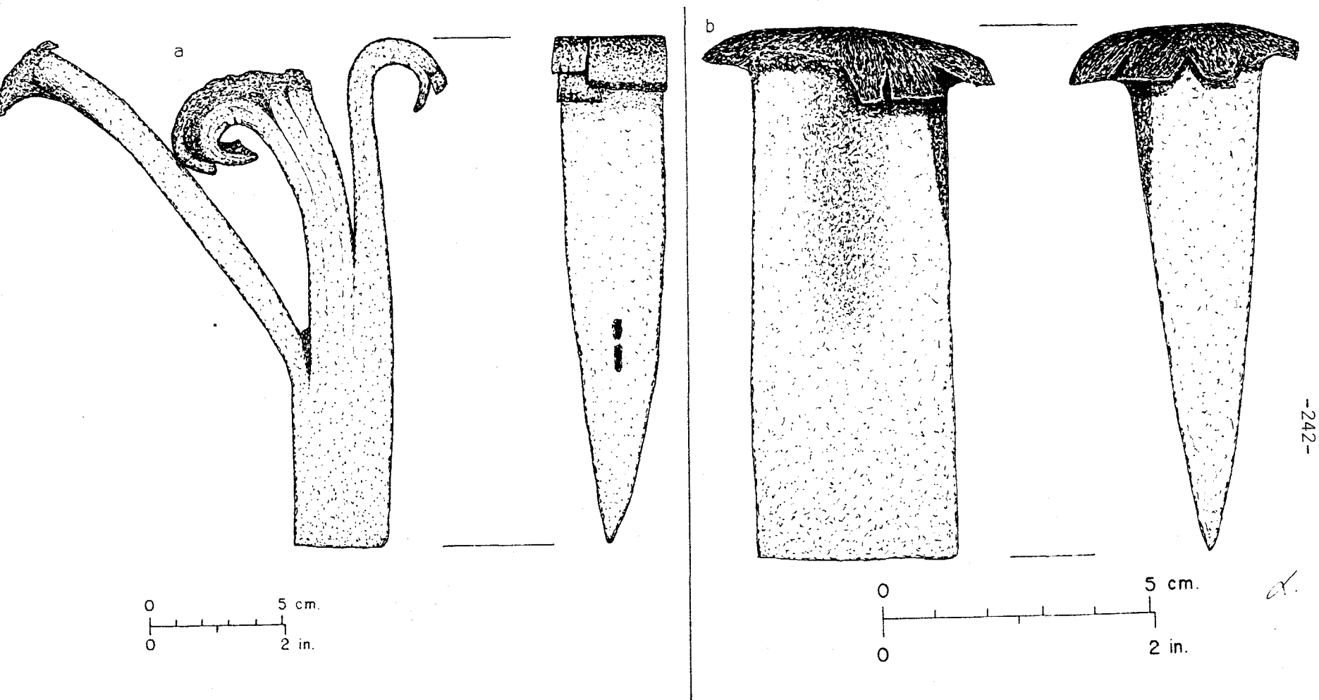
Fig. 128 -- Wedges from F523: a). wedge (FOVA 27974) and b). wedge (FOVA 27819).
