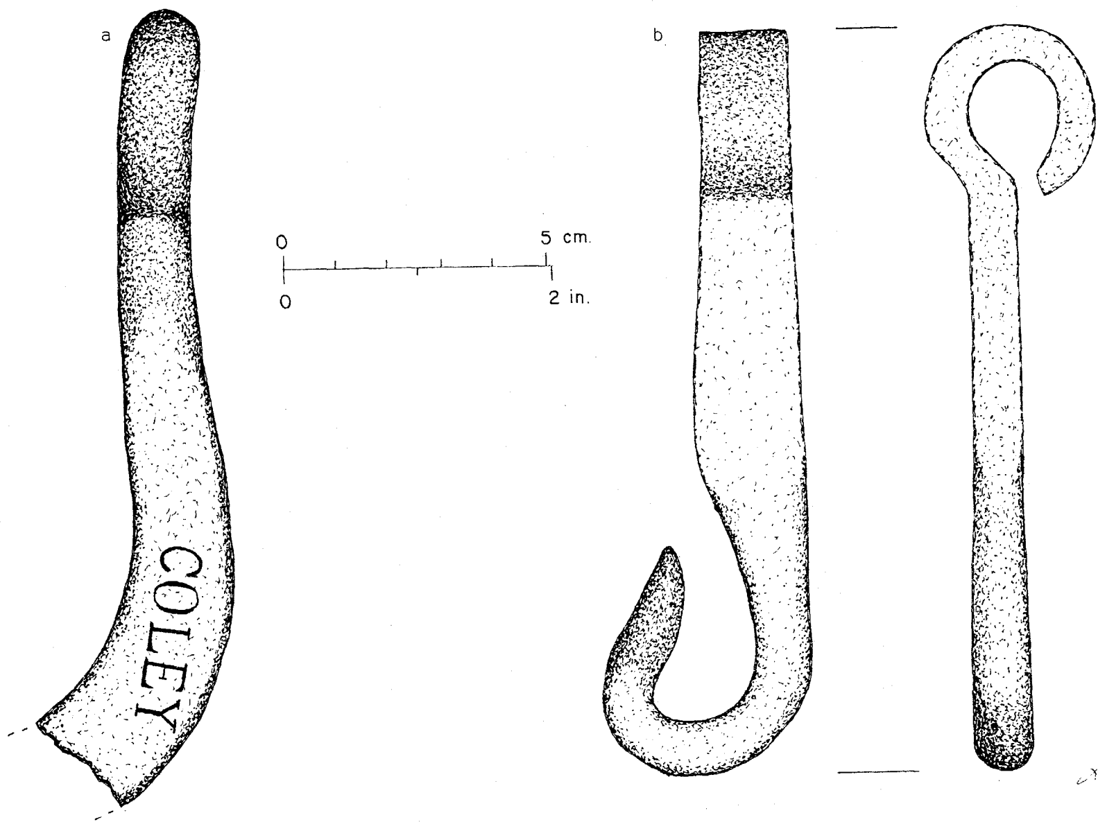
Fig. 148 -- Hooks from F523: a). "COLEY" hook fragment (FOVA 28250) and b). hook (FOVA 28342).
