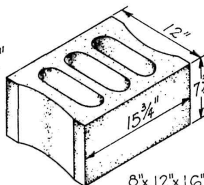
8" x 12" x 16"
