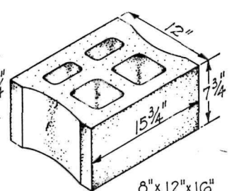
8" x 12" x 16"
