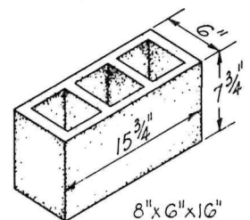
8" x 6" x 16"
